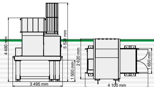
Einwellenbrecher Typ 492 Одновалный измельчитель Тип 489
